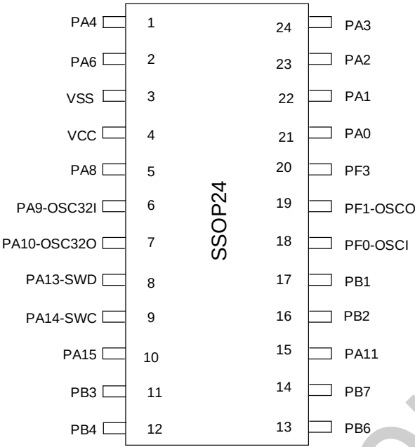
图 3-5 SSOP24 Pinout3 PY32F032E3xM7 (Top view)
